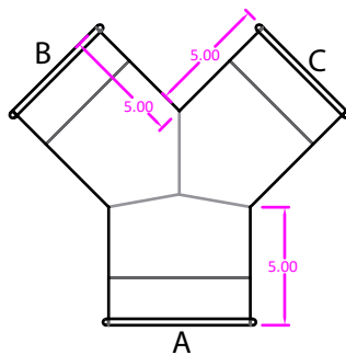
True Y Branch
